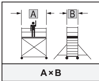
Largura plataforma x anchura bastidor
