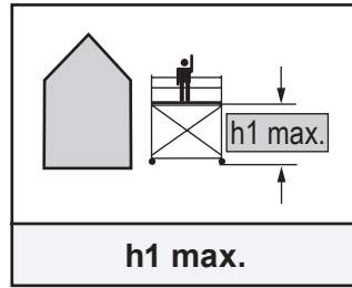
h1 max. Altura máxima admissível do andaime, quando utilizado fora de edifícios
